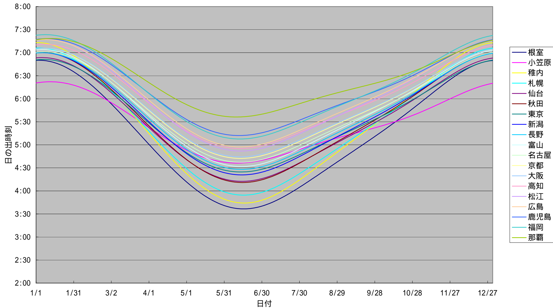
日の出時刻の年間推移
